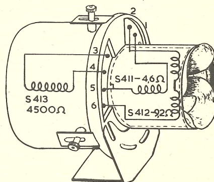
Deflectie-juk GK 565 22
