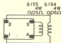
Antennespoel GK 565 24
